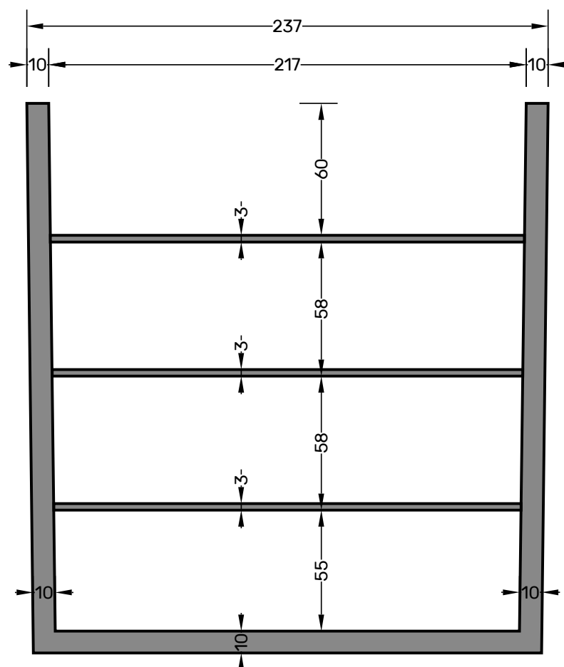
Coupe B-B
