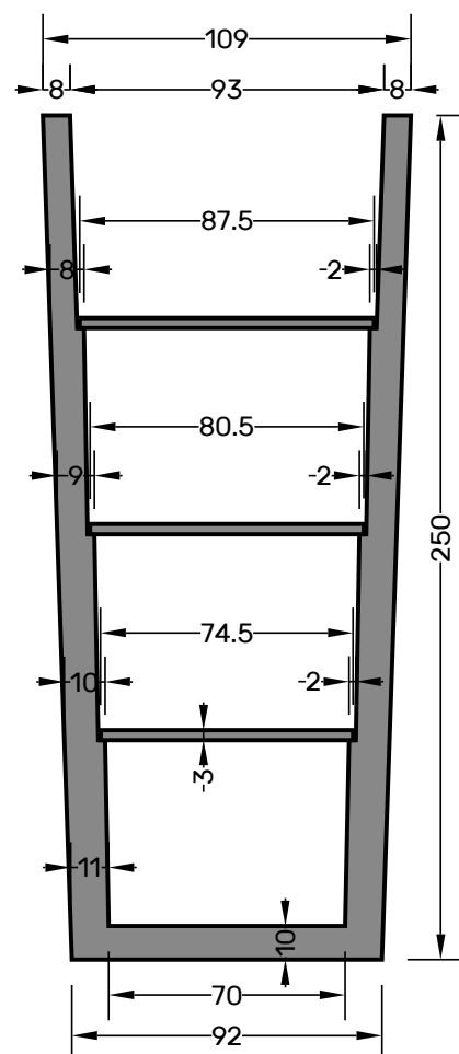
Coupe A-A
